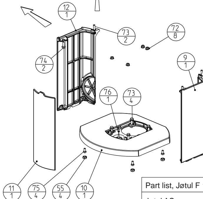
Jøtul F 136
