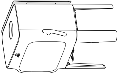
Jøtul F 305 LL (Långa ben)
