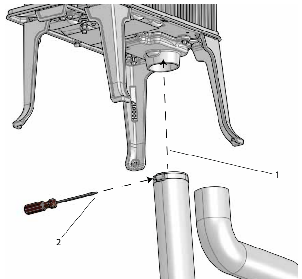
Kuva 10 Raitisilmaliitännän asentaminen
