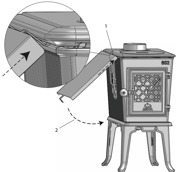
Fig. 4 Montera skärmplatta (tillval)
