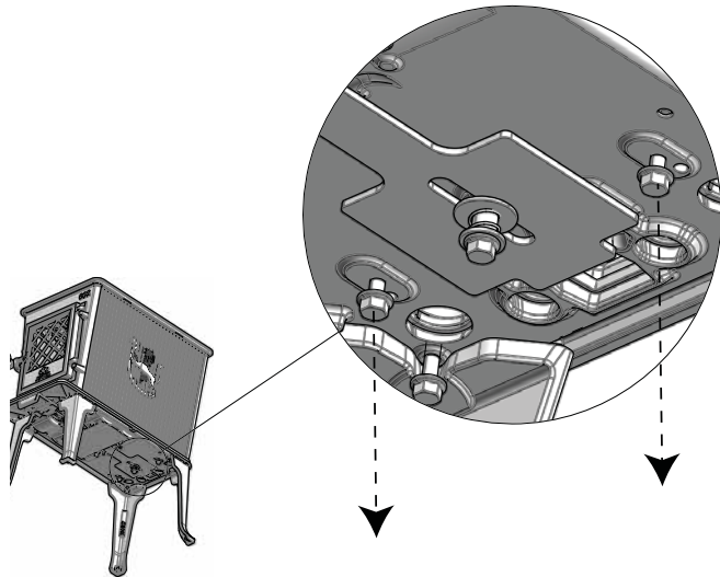
Kuva 7 Raitisilmaliitännän kannen ruuvien irrottaminen
