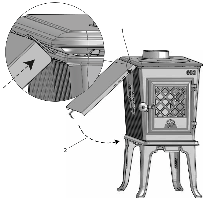
Fig. 4 Montere skærmlade (tillægsudstyr)
