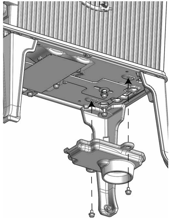
Kuva 9 Raitisilmaliitännän kannen kiinnittäminen
