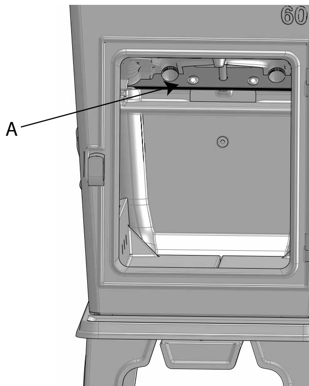
Kuva 24 Takalevyä vasten olevan tiivisteen korvaaminen
