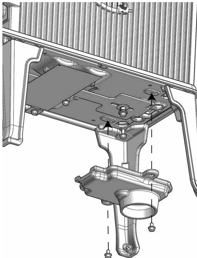
Fig. 9 Montering av uteluftsdeksel
